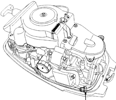
Filtro de combustível
