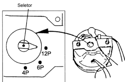
Tacômetro
