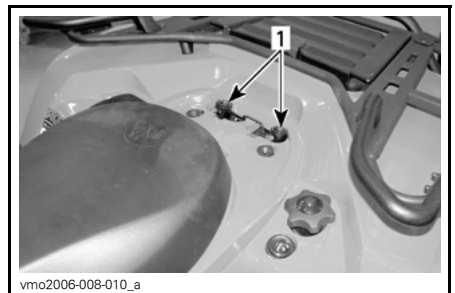
1. Bohrungen für Positionierstäbe des Beifahrersitzes
