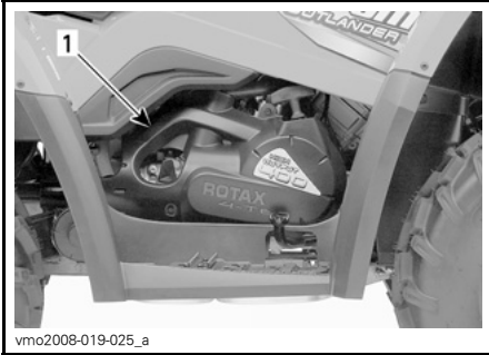
1. Motorabdeckung
