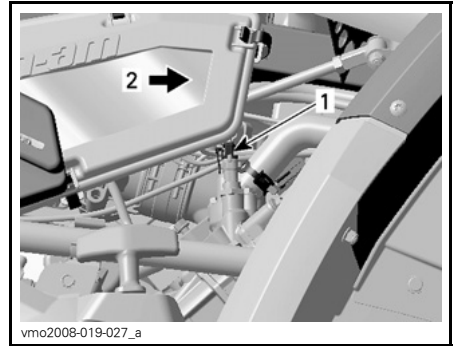
1. Temperatursensor 2. Fahrzeugvorderseite
