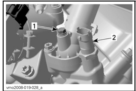
1. Abflussschraube 2. Motortemperaturfühler
