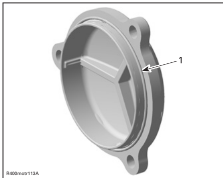
1. O-Ring montiert
