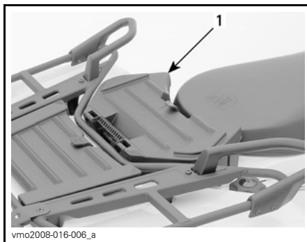
1. Tragbarer Gepäckbehälter
