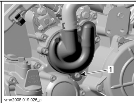
1. Kühlmittelablassschraube
