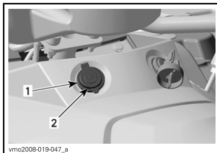
1. 12-Volt-Stromausgang 2. Schutzdeckel
