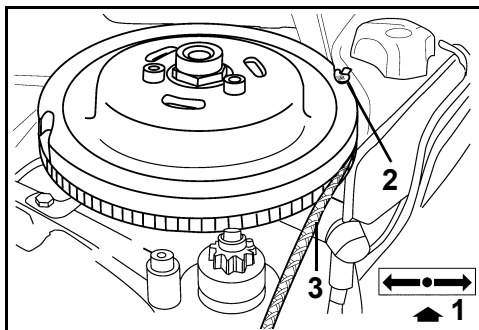
1. FOLLE 002022 2. Nodo 3. Fune nella scanalatura del volano
