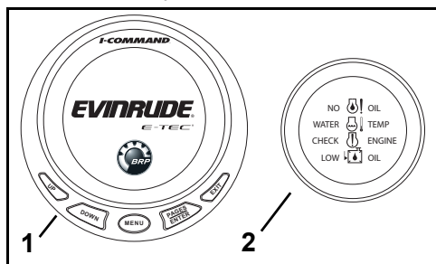
1. Indicatore digitale tipico I-Command
