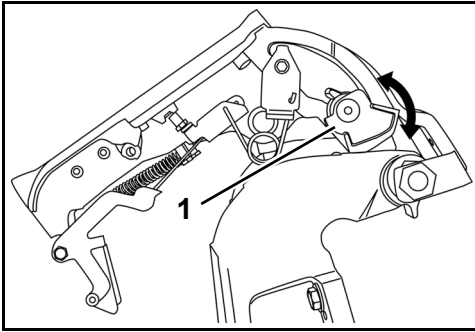
1. Leva di blocco di inclinazione: posizione di blocco
