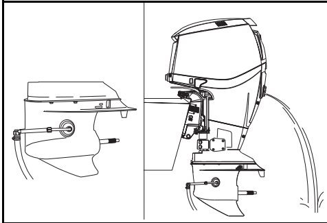
1. Dispositivo di risciacquo 2. Flusso d'acqua
