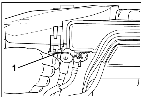
1. Fusibile 002019
