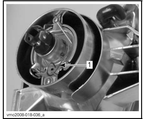
TYPBILD 1. Fästklämma
