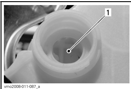
1. Kylvätska här
