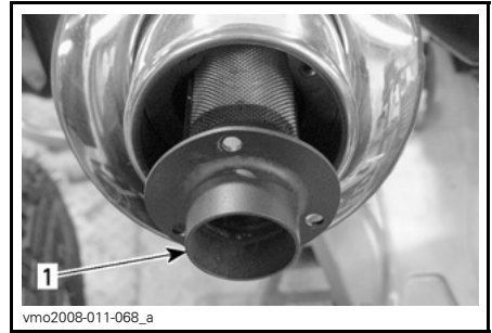
QUITAR 1. Supresor de chispas
