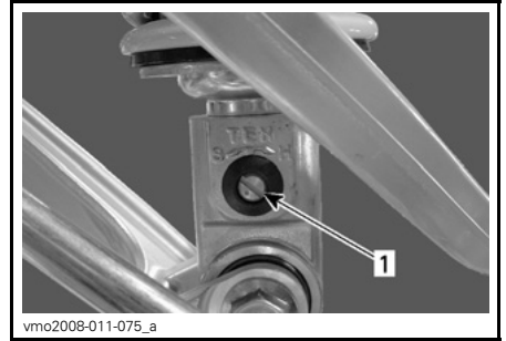
1. Ajustador del rebote (destornillador plano)
