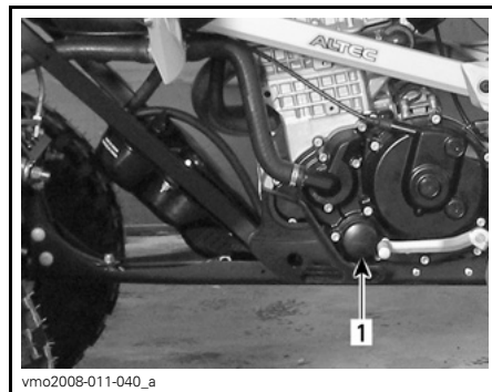
LINKE SEITE DES FAHRZEUGS 1. Ölfilter
