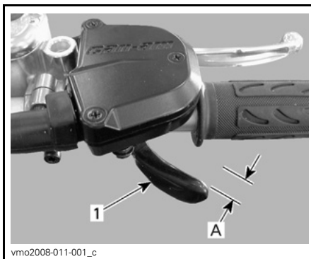
1. Gashebel A. 2 bis 4 mm
