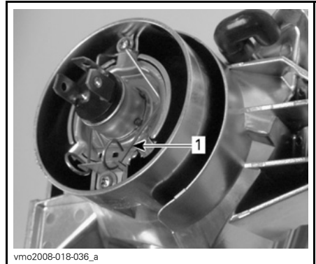
TYPISCH 1. Halteklammer
