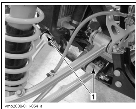
TYPISCH — UNTERER QUERLENKER
