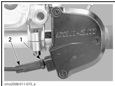
1. Kontermutter 2. Regler
