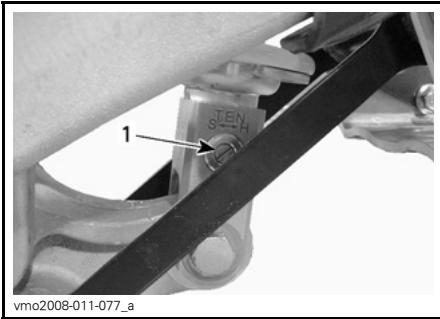
1. Rückstossregler (flacher Schraubenzieher)
