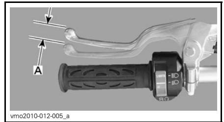
KUPPLUNGSHEBEL — RICHTIGE EINSTELLUNG A. 10 mm bis 15 mm
