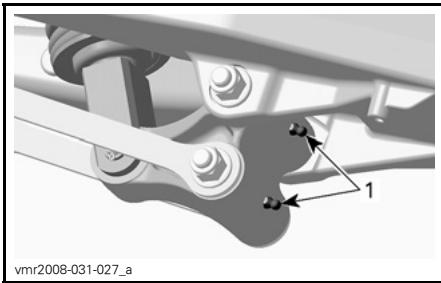
GASREGELAAR 1. Smeerfittingen
