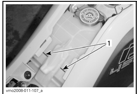
KOELMIDDELRESERVOIR 1. Peilmerktekens
