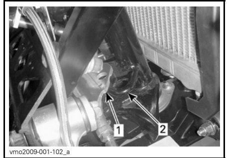
1. Chassisbeugel 2. Stuurkolombeugel
