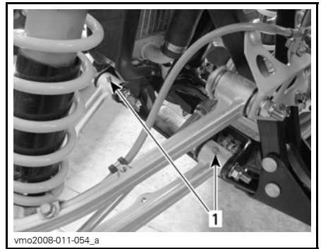
TYPISCH — ONDERSTE WIELDRAAGARM 1. Smeerfittingen
