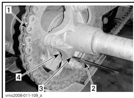
1. Aandrijfketting 2. Punt schroevendraaier (gereedschapsset) 3. Kettingwielnaaf 4. Excenterasbehuizing
