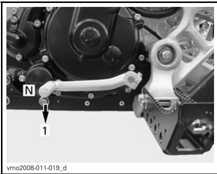
1. 1 e versnelling
