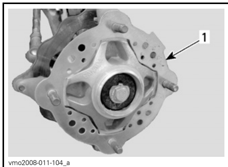
VOORWIEL
