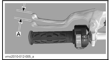
TYPISCH — NOMINALE SPELING KOPPELINGSHENDEL A. 10 mm tot 15 mm
