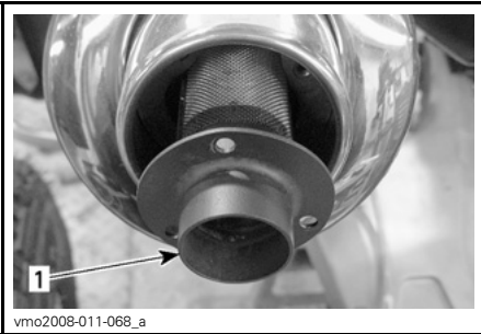
1. Vonkafleider
