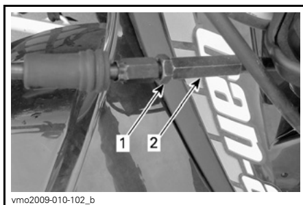
1. Borgmoer 2. Afstelschroef
