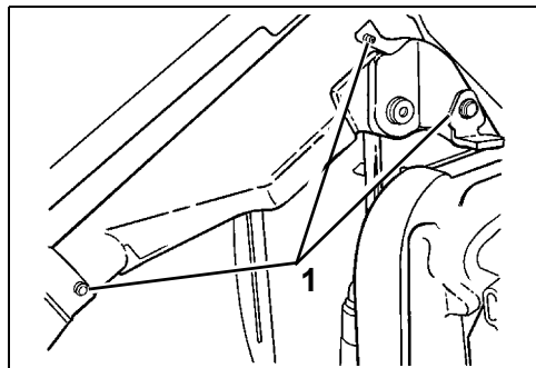
1. Pontos de lubrificação da alavanca de inclinação e do suporte giratório (anualmente) DR31329
