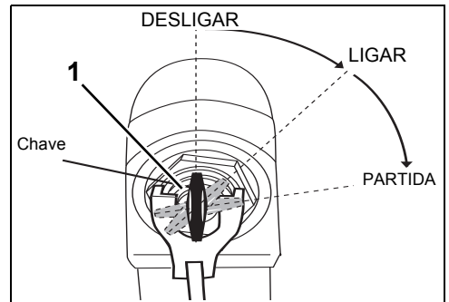
1. Interruptor da chave, posição OFF (desligado) 007072
