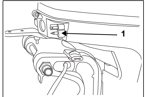
1. Connecteur de carburant (typique)
