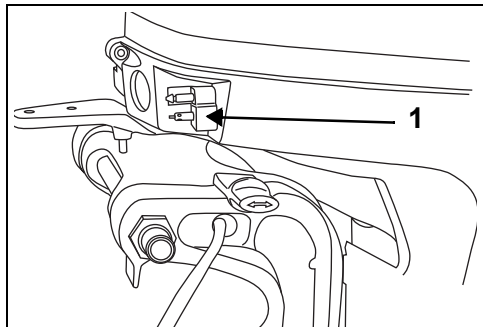
1. Connecteur de carburant (typique)
