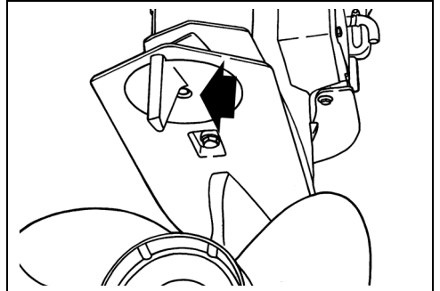
Trimmflossenschraube
