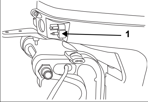
1. Kraftstoffanschluss (typisch)
