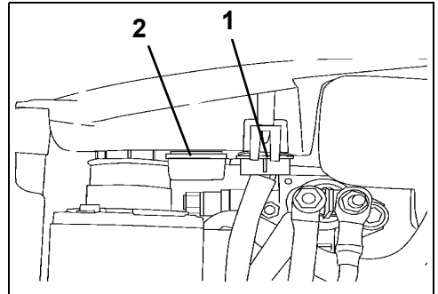
1. Sicherung 2. Ersatzsicherung
