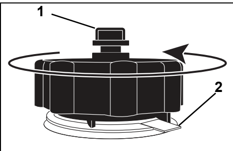
1. Entlüftungsschraube 2. Druckentlastungszunge
