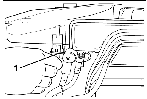
1. Sicherung 002019
