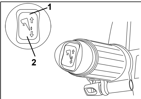
1. Trimm-/Kippschalter nach oben 005107 2. Trimm-/Kippschalter nach unten
