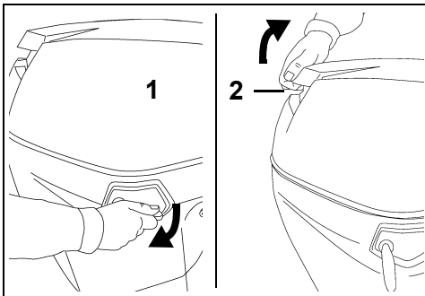
1. Verriegelung der Motorabdeckung 002015 2. Kippgriff 002016
