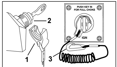
1. Klemme DR6819 2. Motor-Hauptschalter/Zündschalter DR5592 3. Sicherheitsleine
