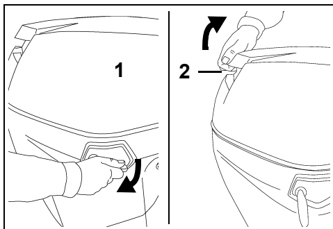
1. Motordekselsperre 2. Tilthendel
