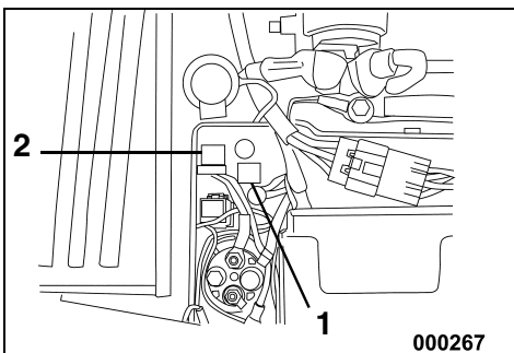
1. Fusible 2. Porte-fusible de rechange
