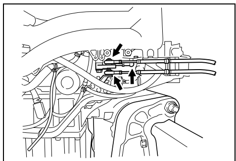
1. Tringlerie d'accélération et de commande de sens de marche
