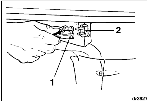
1. Raccord de flexible de carburant 2. Raccord de carburant
