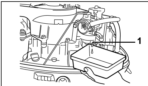
1. Vergaser-Ablassschraube
