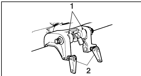
1. Gaslänksystem
