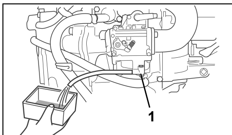
1. Förgasarens tömningsskruv
