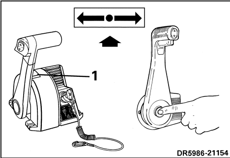
1. Κουμπί επιλογής υψηλών στροφών ρελαντί
