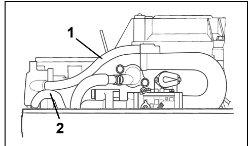
1. Σωλήνας εξαγωγής αναθυμιάσεων 2. Σωλήνας παροχής καυσίμου
