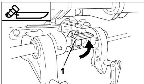
1. Leva di blocco ribaltamento in posizione TILT
