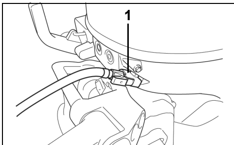
1. Flessibile di alimentazione al connettore di alimentazione
