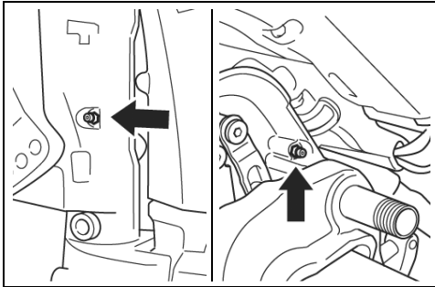
Staffa dello sterzo
