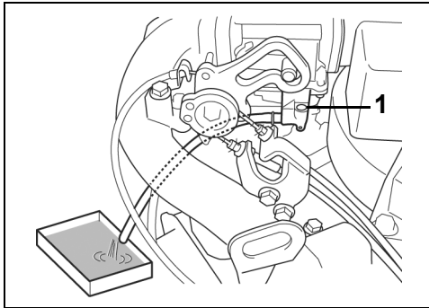
1. Vite di spurgo del carburatore
