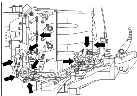
Articulação do acelerador e câmbio
