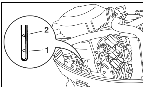
1. Toevoegen 2. Vol
