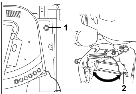
1. Stuurfrictie-regelschroef 2. Stuurfrictiehendel
