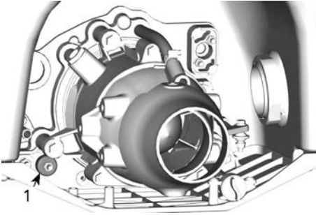
1. Plassering av offeranode
