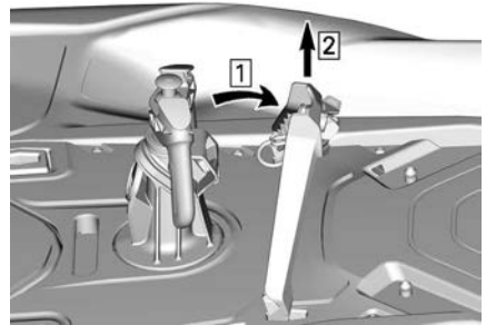
1. Kippträger 2. Hebeträger
