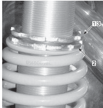
ТИПОВОЙ ВАРИАНТ – АМОТИЗАТОР С РЕГУЛИРОВОЧНОЙ РЕЗЬБЕЙ
