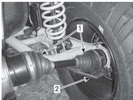
ТИПОВОЙ ВАРИАНТ — ЗАДНЯЯ ЧАСТЬ МОТОВЕЗДЕХОДА
