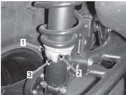
ТИПОВОЙ ВАРИАНТ – АМОТИЗАТОР С РЕГУЛИРОВОЧНЫМ КУЛАЧКОМ
