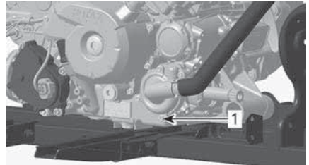
ТИПОВОЙ ВАРИАНТ — ДВИГАТЕЛИ 570/650/850
