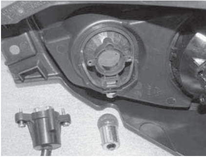
TYPISCH - HINTERE BLINKERLAMPE
