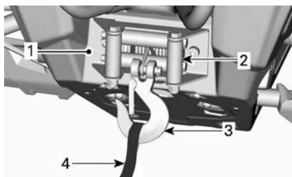
1. Guincho 2. Guia do cabo 3. Gancho do guincho 4. Alça do gancho
