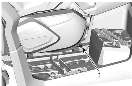
1. Reservatório de drenagem da CVT
