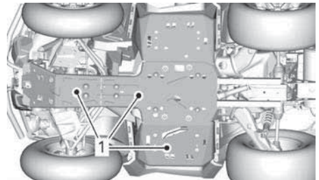
1. Schutzplatten
