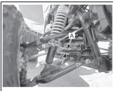
ПЕРЕДНЯЯ ПОДВЕСКА
