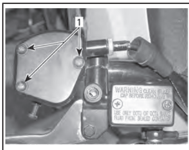
1. Выверните винты
