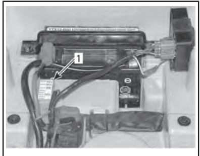
1. Porte-fusible
