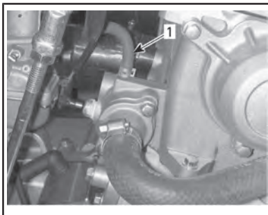
1. Flexible de dérivation
