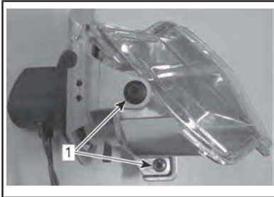
1. Vis à desserrer
