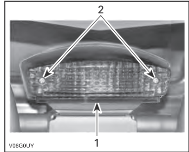
1. Lentille 2. Vis
