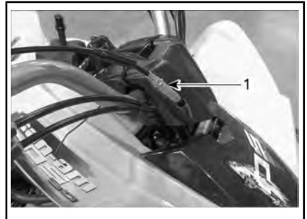
JUSTERING FRA GASSHÅNDTAK TIL TURTALLSBEGRENSERBOKS
