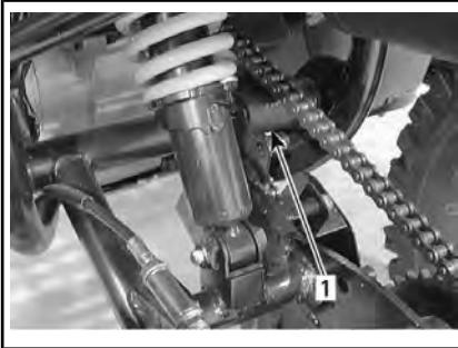
1. Drivkjederulle
