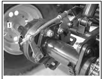
1. Bremsevaierjustering
