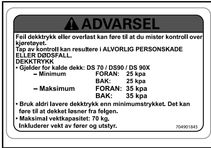
DEKAL 4 – TYPEBILDE
