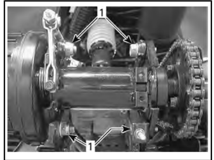
TYPEBILDE – BAKAKSEL
