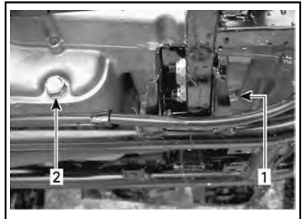
BOUCHON DE VIDANGE — CÔTÉ GAUCHE DU MOTEUR
