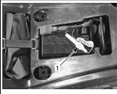
1. Porte-fusible
