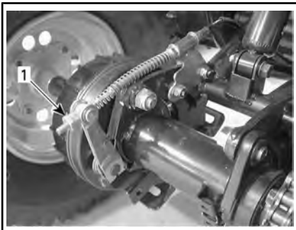
1. Dispositif de réglage de câble de frein
