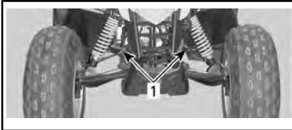
1. Vis de réglage sur les câbles
