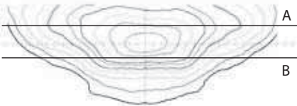
TYPISCHE LICHTBUNDEL VAN KOPLAMPEN OP TESTOPPERVLAK
