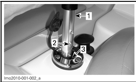
1. Tige du feu de poupe 2. Tête de vis de la tige 3. Orifice de fixation du logement
