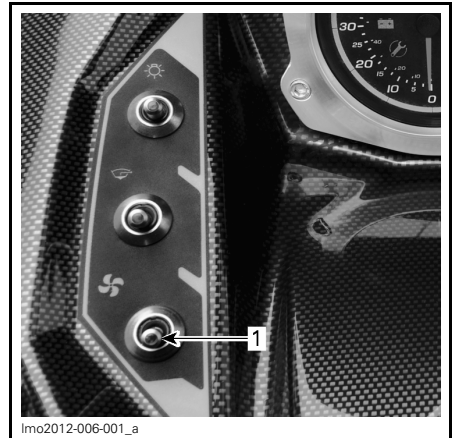
INTERRUPTEUR DU VENTILATEUR DE CALE 1. Interrupteur du ventilateur de cale
