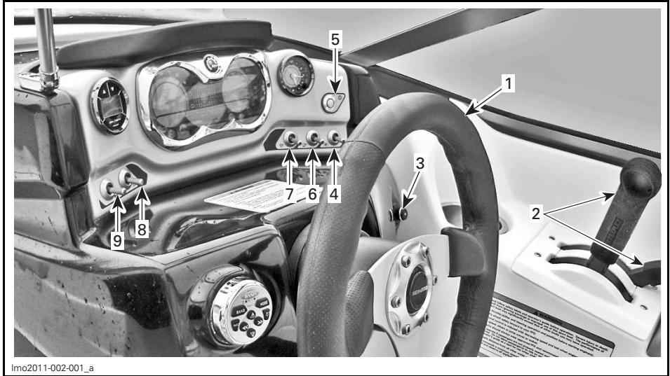
VUE DU COCKPIT
