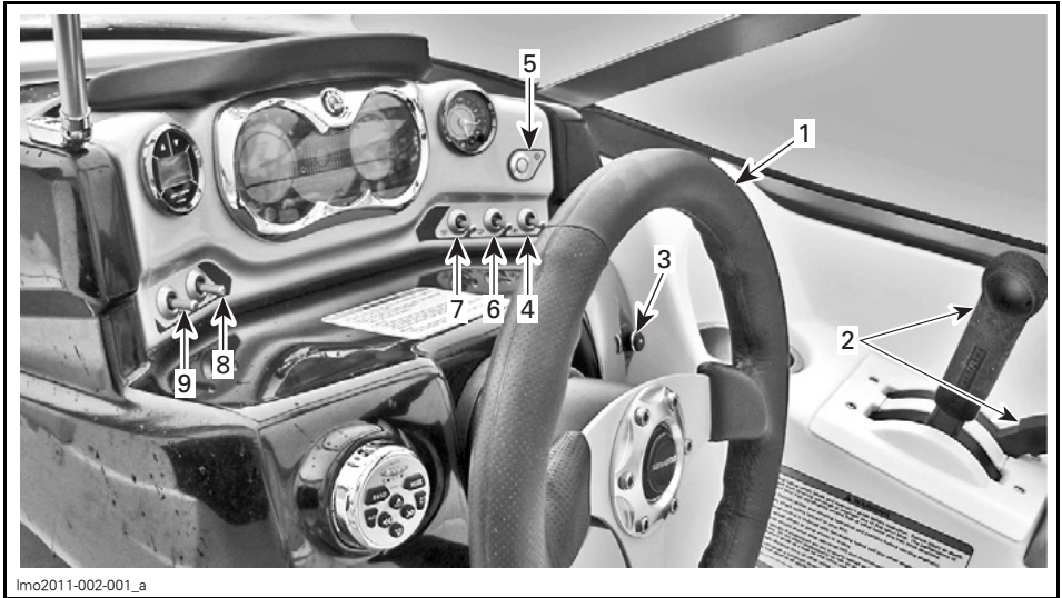
COCKPIT-ANSICHT
