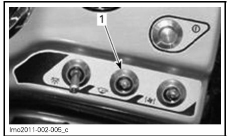
1. Schalter für Bilgepumpe
