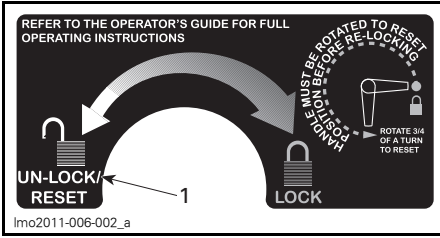
1. ENTRIEGELUNGS-/RÜCKSTELL-Position (Backbordseite)
