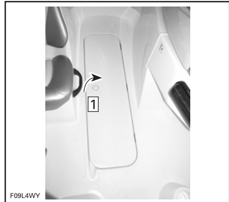
TYPISCH Schritt 1: Verschluss hochziehen und Abdeckung abheben
