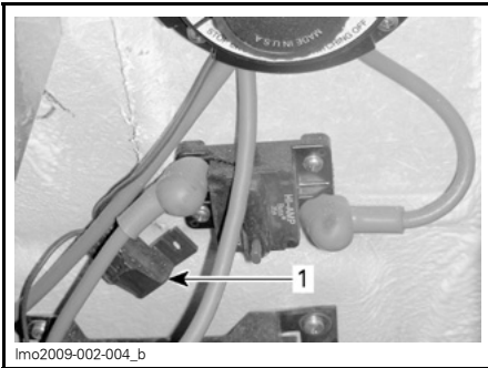
1. Sicherung der automatischen Bilgenpumpe
