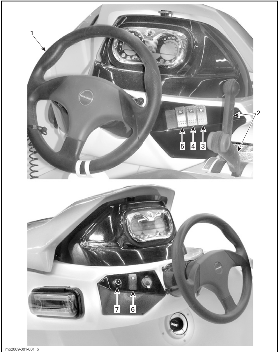
VISTA DO COCKPIT (POSTO DE COMANDO)
