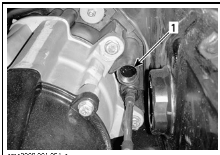
1. Conexão de lavagem — localização pode diferir
