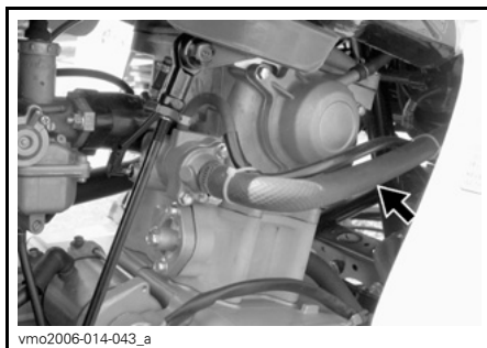
LOCAL DA PINÇA PARA MANGUEIRA
