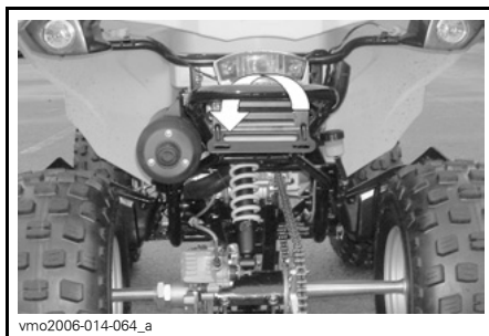
TÍPICO – LOCAL DA CORREIA DO PÁRA-CHOQUE TRASEIRO
