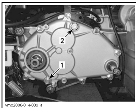
1. Tampão de drenagem da caixa de câmbio 2. Tampão de abastecimento da caixa de câmbio
