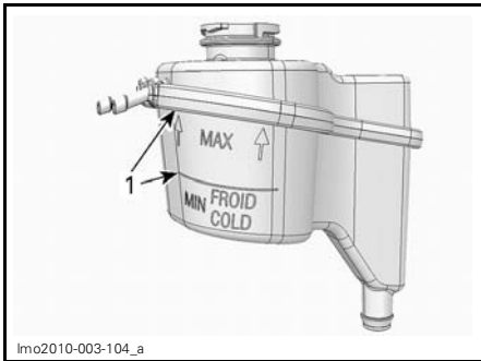
1. Niveau entre les marques alors que le moteur est froid
