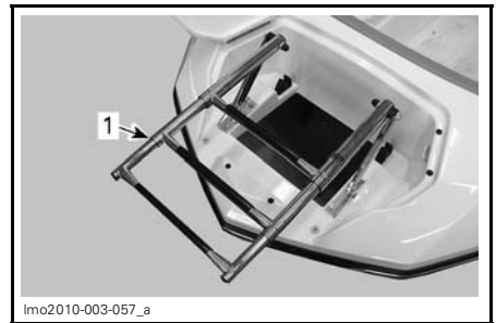
1. Échelle déployée
