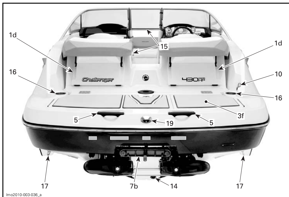
VUE D'EN ARRIÈRE
