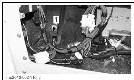
1. Porte-fusibles de la radio
