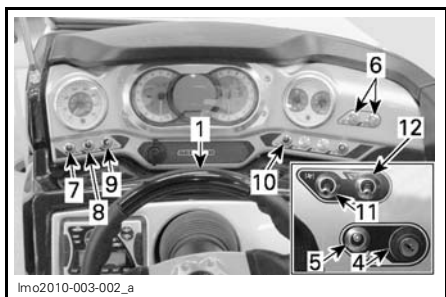
PARTIE SUPÉRIEURE DE LA CONSOLE DU CONDUCTEUR
