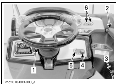
PARTIE INFÉRIEURE DE LA CONSOLE DU CONDUCTEUR
