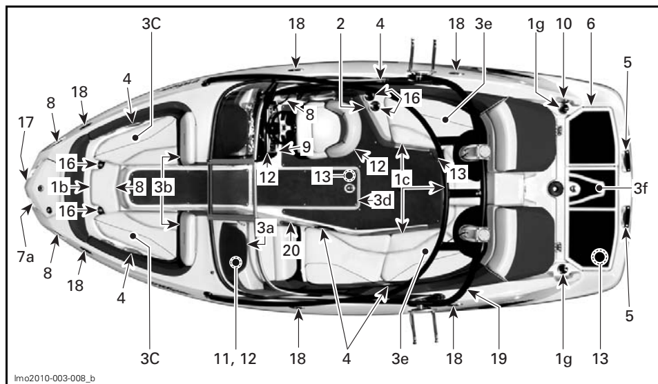
VUE D'EN HAUT
