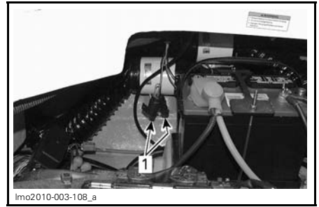
1. Porte-fusibles de ventilateur
