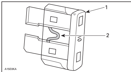
1. Fusible 2. Vérifier si le filament est fondu
