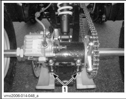
TYPISCH 1. Borgbouten kettingspanner
