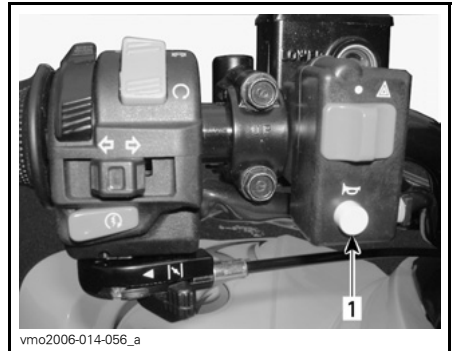
1. Knop voor de claxon
