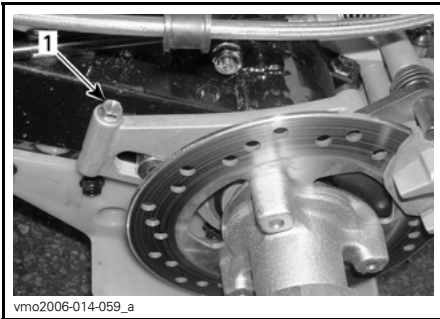
1. Klauwsteunbout
