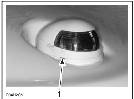
1. Sortir avec précaution à l'aide d'un tournevis
