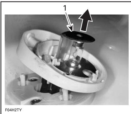
TYPIQUE 1. Soulever et enlever l'ampoule
