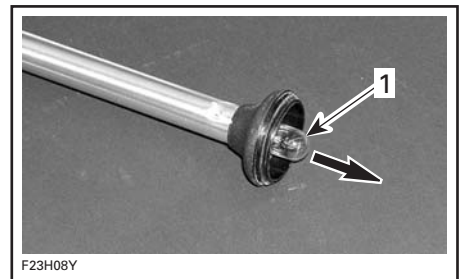
TYPIQUE 1. Enlever l'ampoule
