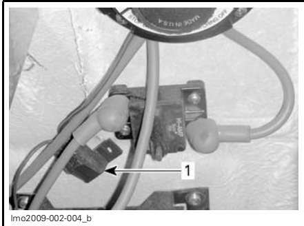
1. Fusible de la pompe de cale automatique
