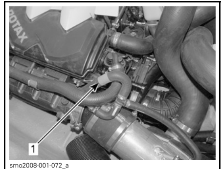
TYPISCH 1. Bringen Sie die Schlauchklemme hier an
