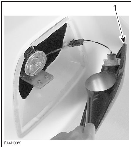
1. Couvercle du feu
