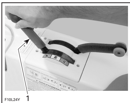
TYPIQUE 1. Levier sélecteur en position de marche avant
