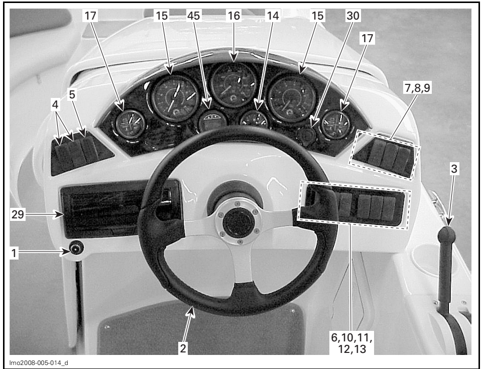
VUE DU COCKPIT
