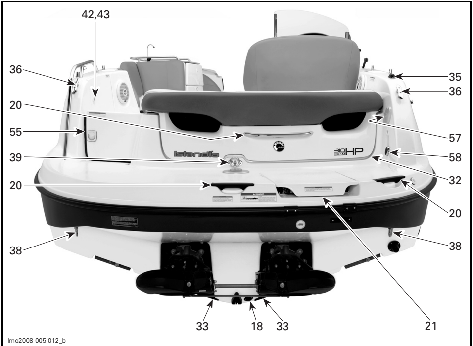
TYPIQUE — VUE DE L'ARRIÈRE
