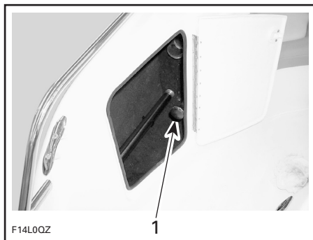
TYPIQUE — FEU DE POUPE DANS LES PINCES DE RANGEMENT
