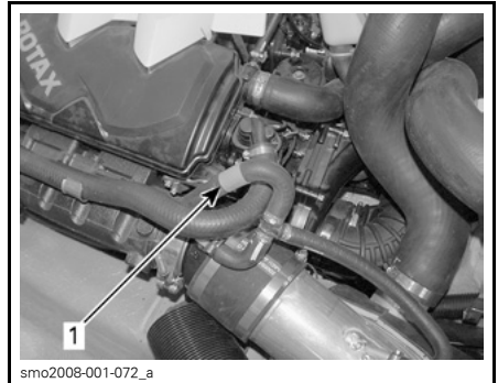
TYPISCH 1. Wasser-Auslassschlauch des Abgaskrümmers
