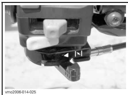
TÍPICO — PALANCA DEL ESTRANGULADOR DE AIRE EN POSICIÓN DE ESTRANGULADOR CERRADO
