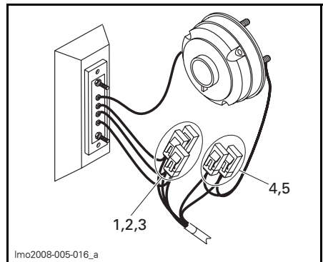
TÍPICO — POR TRÁS DO INTERRUPTOR DE CORTE DA BATERIA
