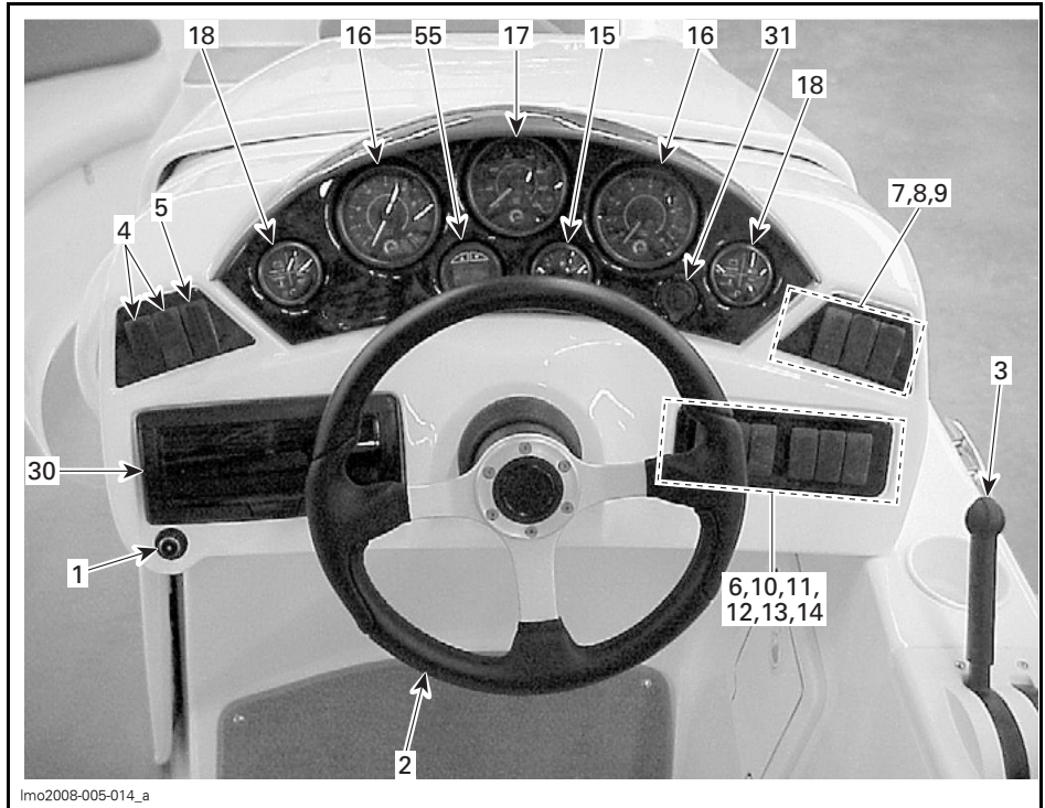
VISTA DO POÇO (COCKPIT)
