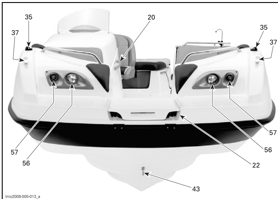
TÍPICO — VISTA FRONTAL
