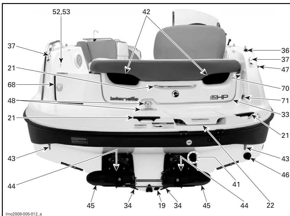
TÍPICO — VISTA TRASEIRA
