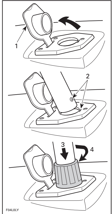
TYPISCH 1. Anheben 2. Schraube in Nut ausrichten 3. Nach unten drücken 4. Drehen zum Verriegeln
