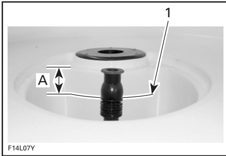
1. Höchster Wasserstand A. 5 cm (1 in) vom oberen Rand
