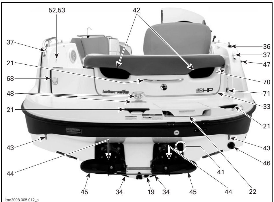
TYPISCH — RÜCK-ANSICHT
