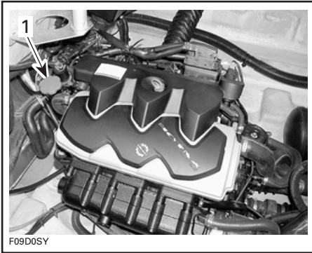
TYPISCH 1. Olievuldop
