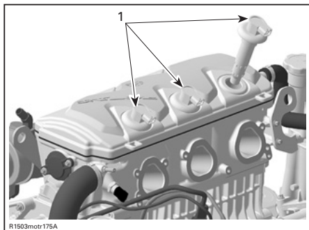
1. Ontstekingsspoelen
