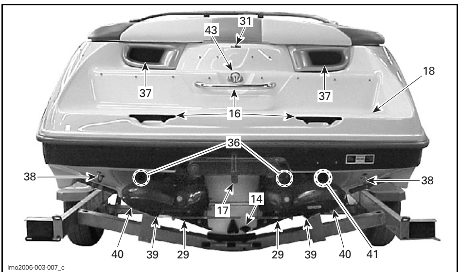
TYPISCH — ACHTERAANZICHT
