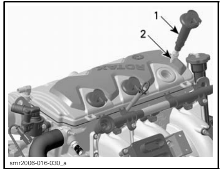
1. Bobine d'allumage 2. Bougie
