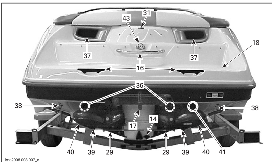
TÍPICO — VISTA POR POPA
