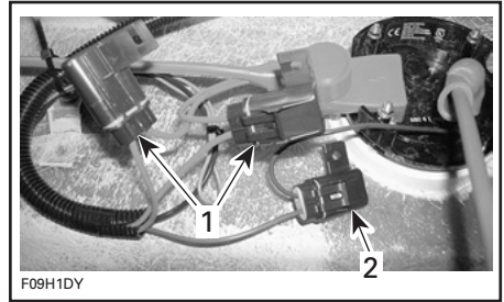
TÍPICO — DETRÁS DEL INTERRUPTOR DE DESCONEXIÓN DE LA BATERÍA
