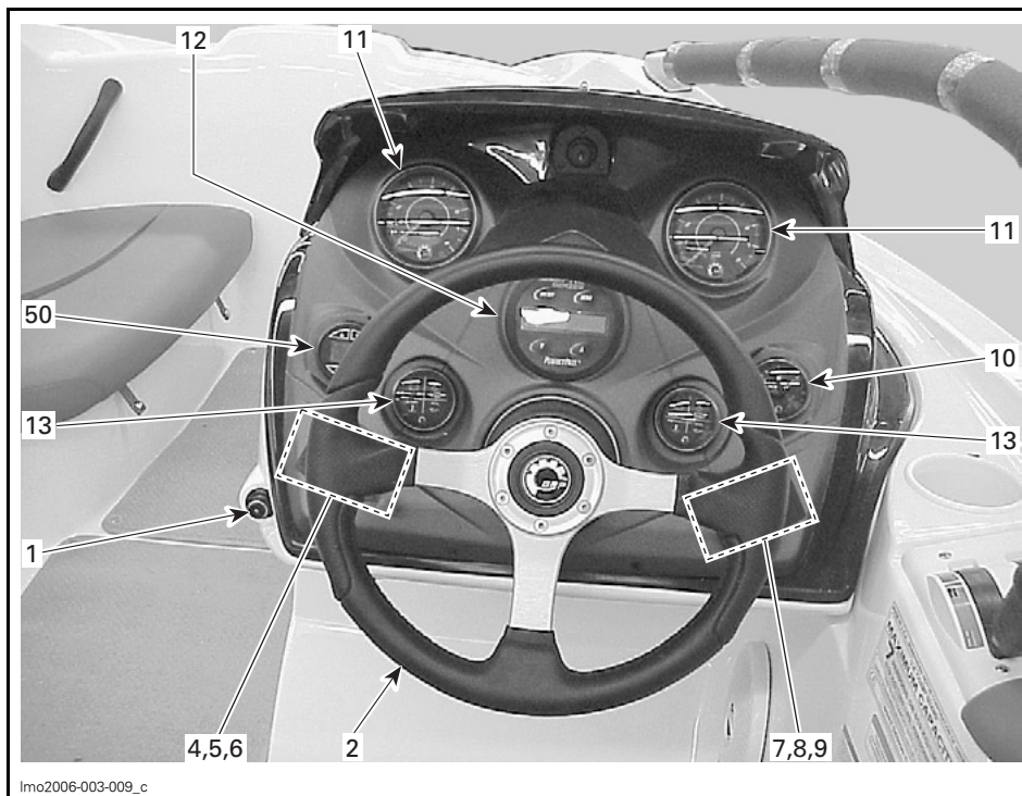
コックピットのレイアウト
