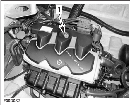
TYPISCH 1. Ölmesstab
