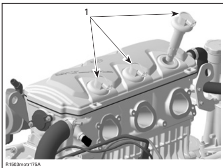
1. Zündspulen
