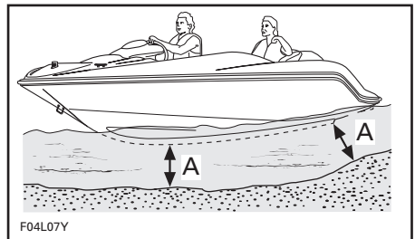
A. Wassertiefe unter dem Rumpf 90 cm (3 Fuß)
