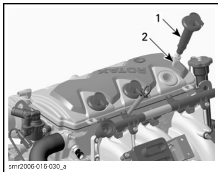
1. Zündspule 2. Zündkerze
