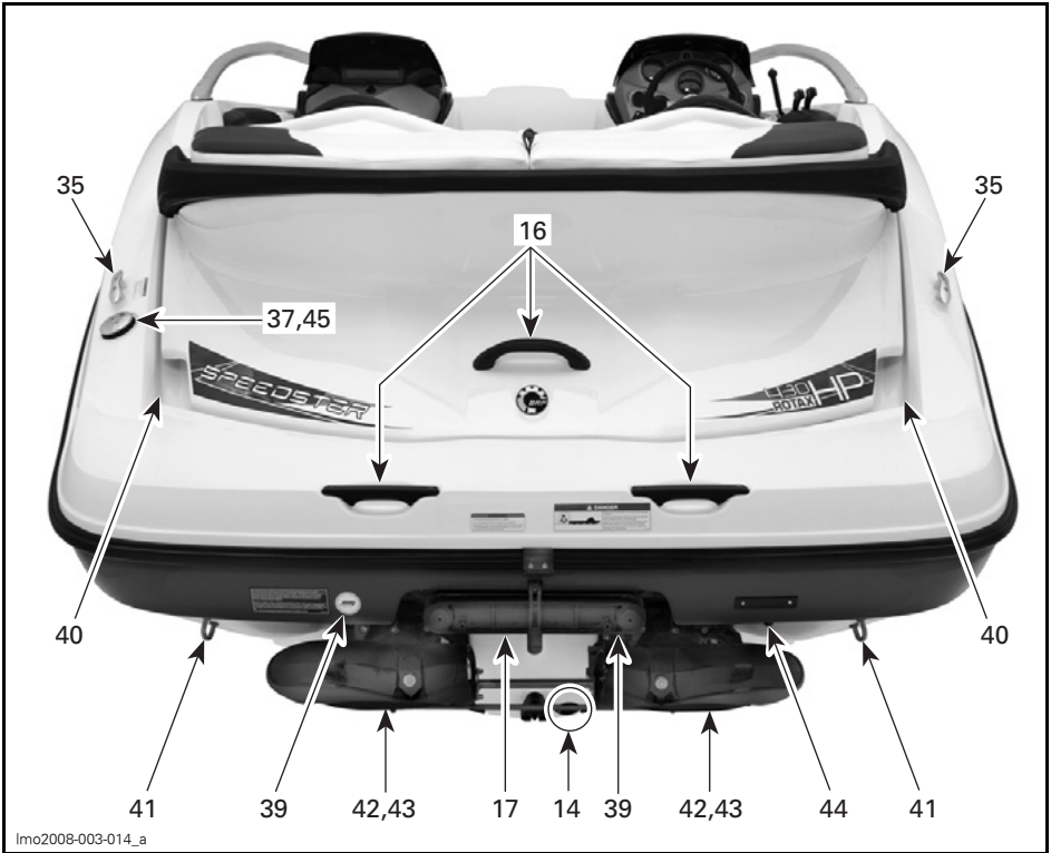
TYPISCH — RÜCKANSICHT
