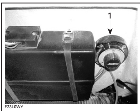
TÍPICO — INTERRUPTOR DE DESCONEXIÓN DE LA BATERÍA PRINCIPAL
